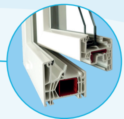
Renforts acier périphériques en fonction des dimensions
